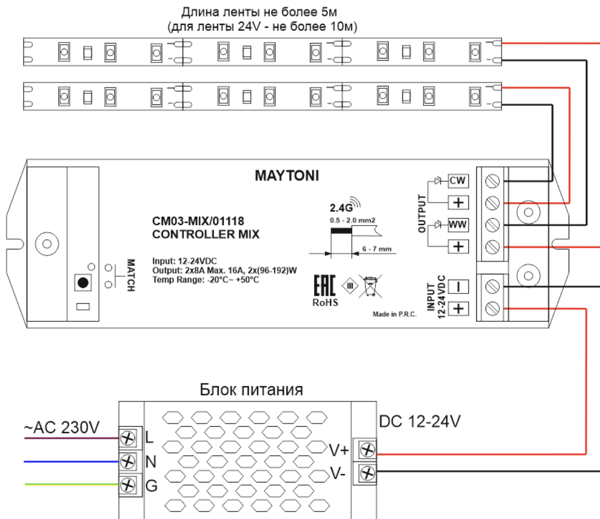
Рис. 2 схема подключения контроллера с использованием монохромной ленты
