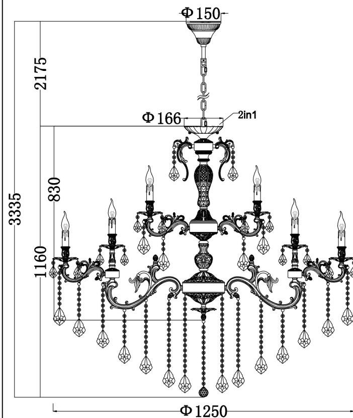
DIA882-PL-30-G 尺寸图
