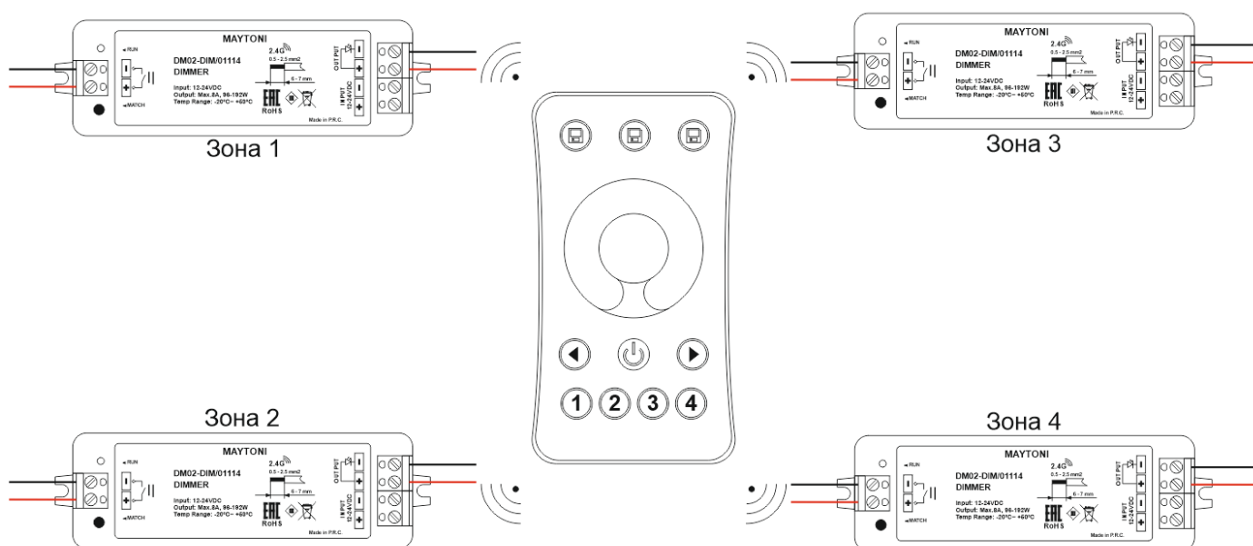
Рис. 3 разветвленная система с многозонным пультом управления
