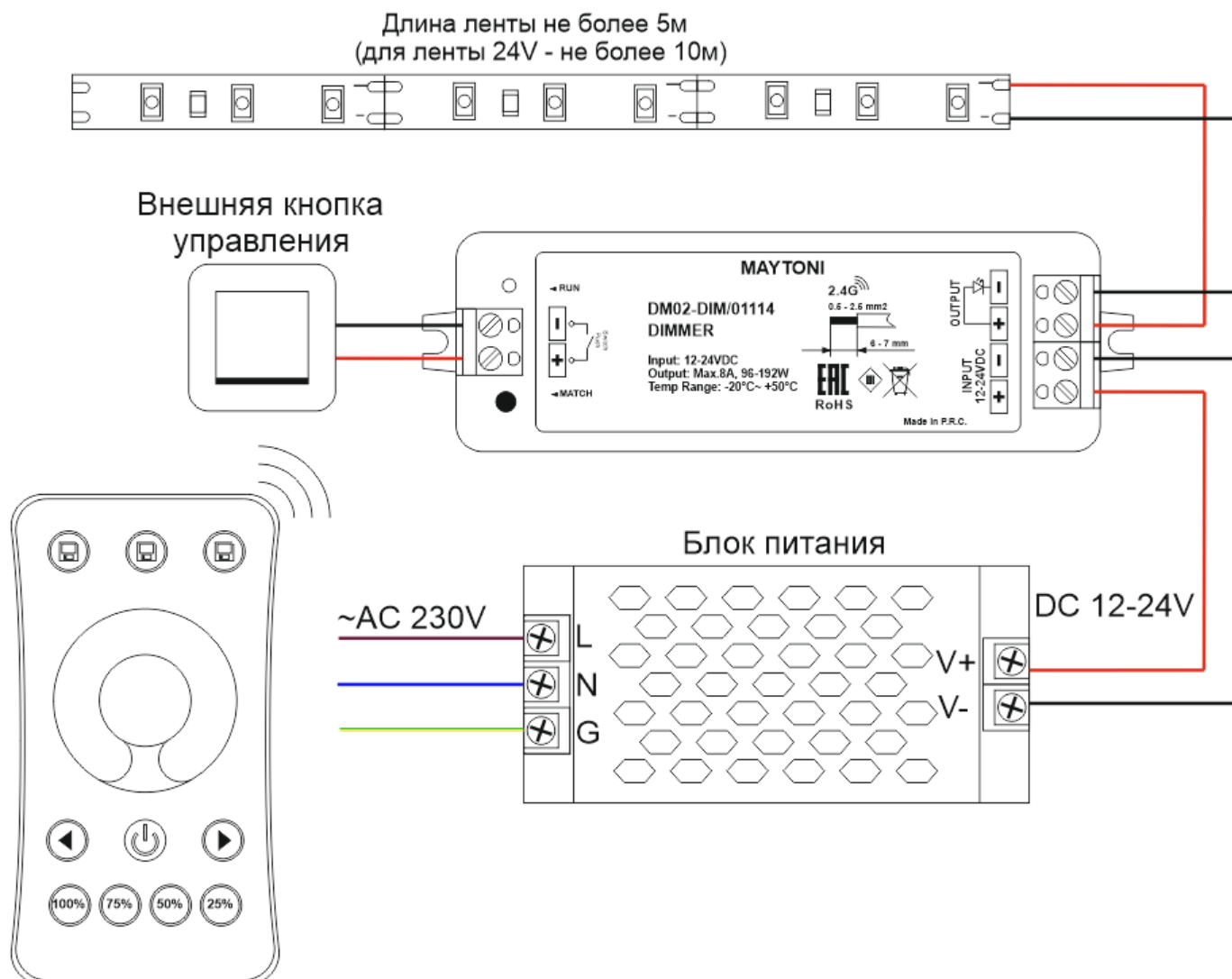
Рис. 1 схема подключения диммера
