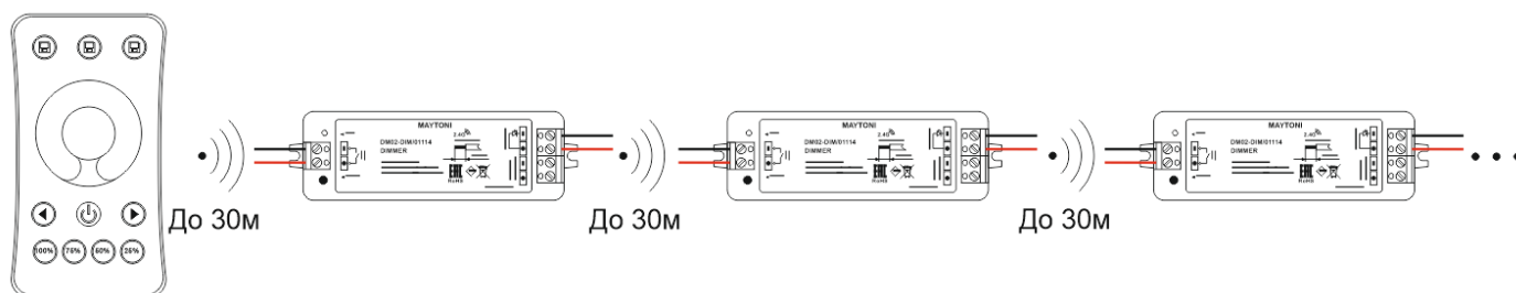
Рис. 2 ретрансляция сигнала между диммерами
