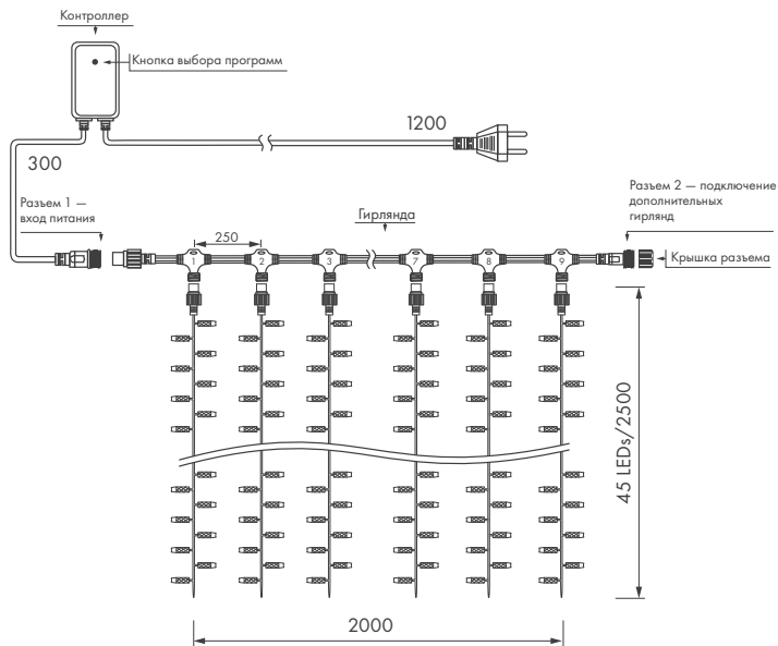
Рисунок 1. Схемы подключения
